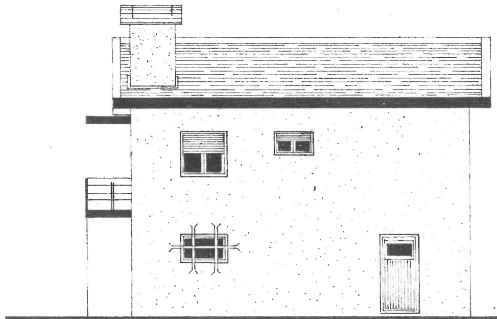
ALÇADO POSTERIOR
