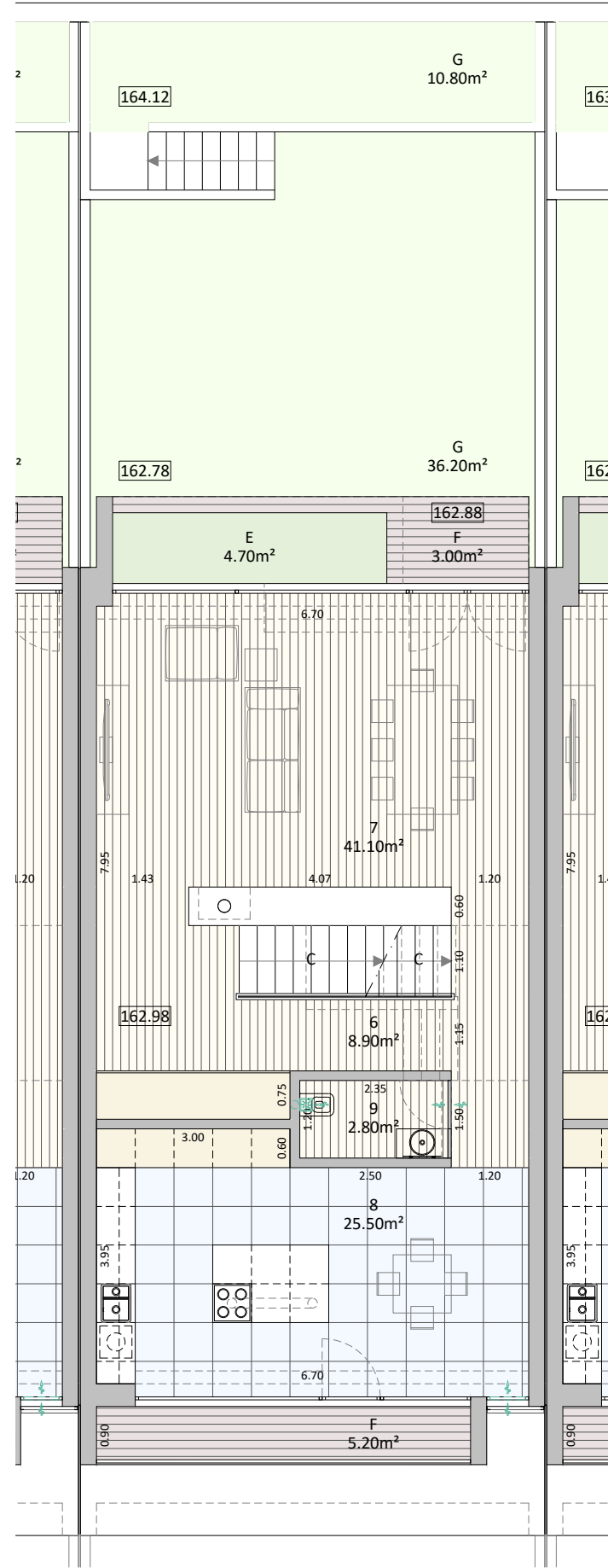
Planta do Piso 1
