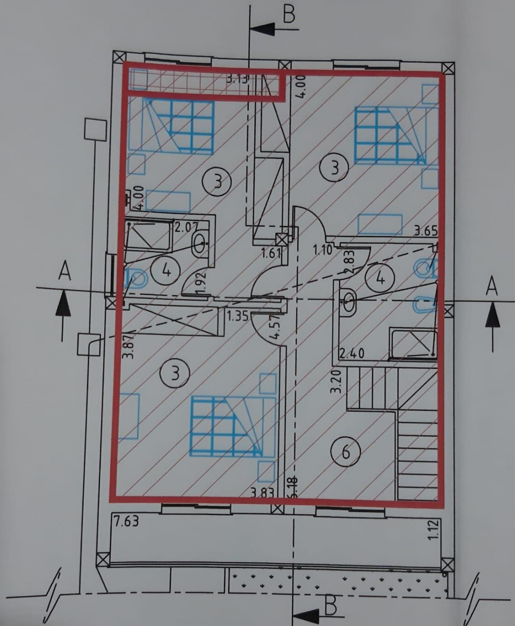
PLANTA DO 1.º ANDAR
