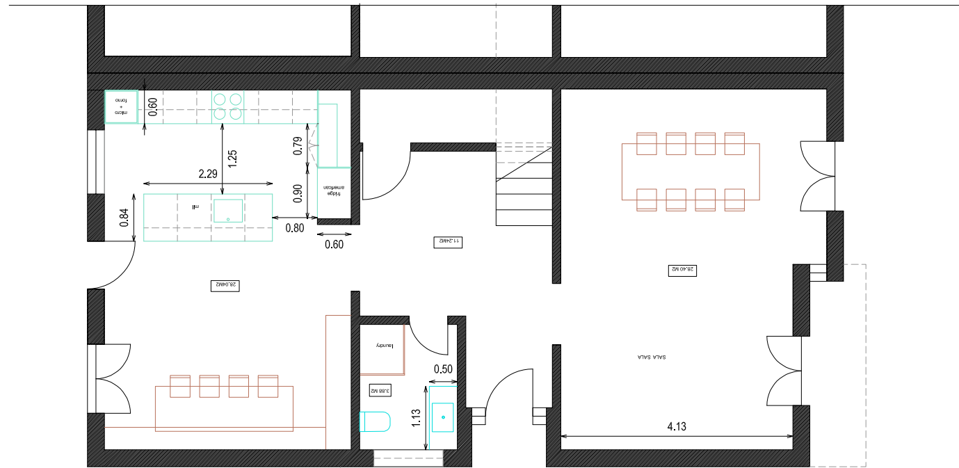
piso 0 - proposto
