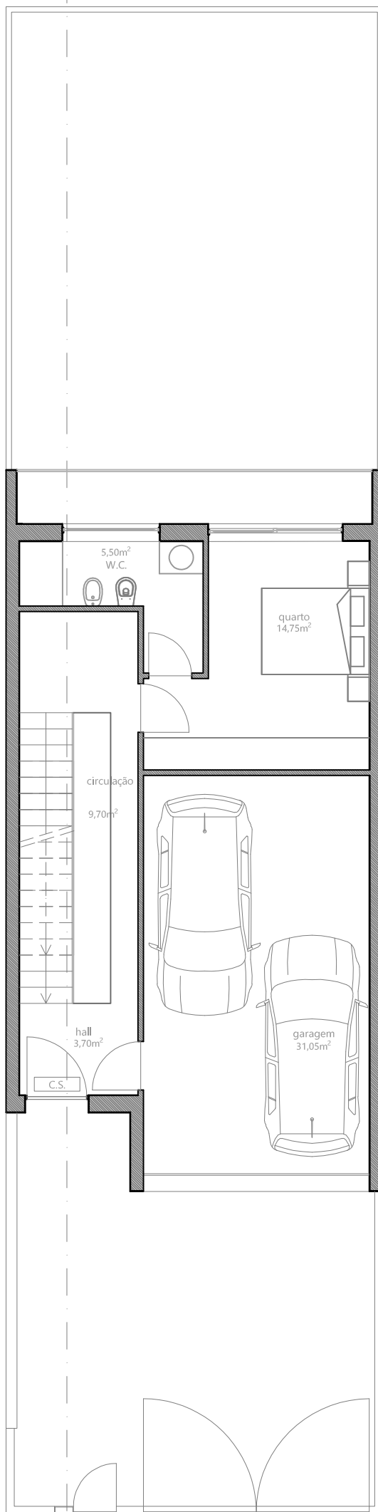
Planta Piso 0
