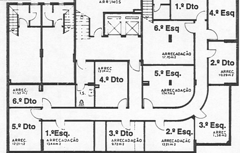
PLANTA DA CAVE
