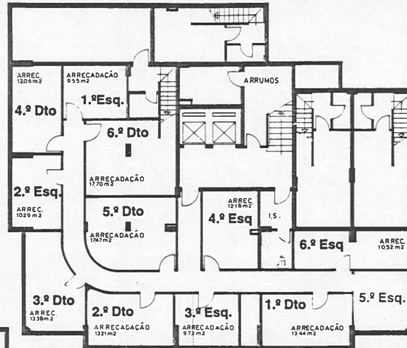
PLANTA DA CAVE
