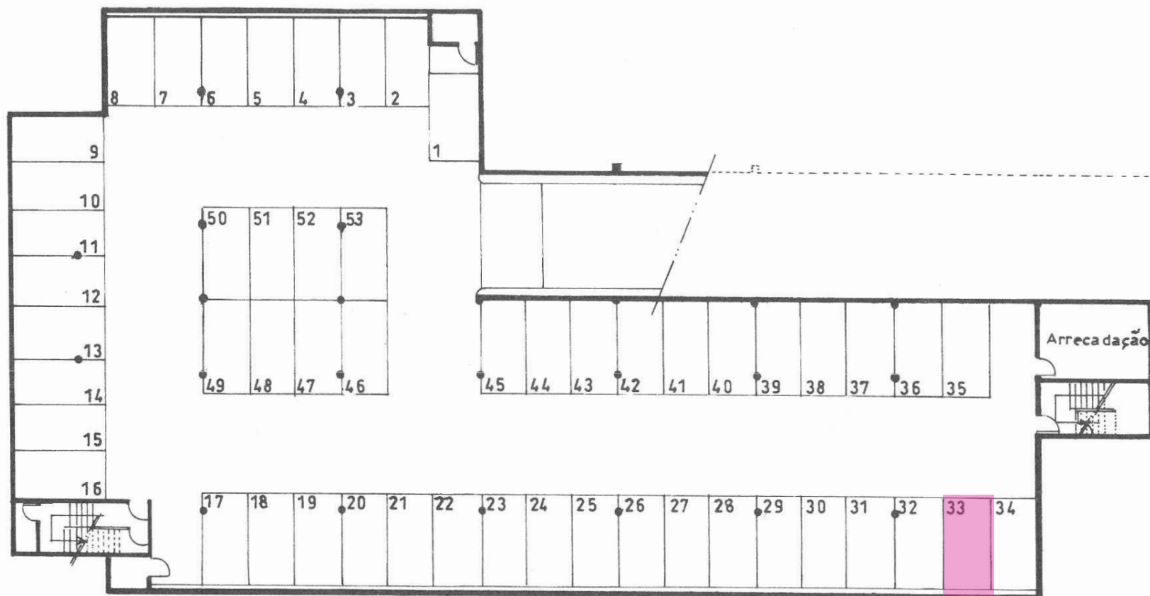
PLANTA DO ESTACIONAMENTO DO PISO - 2
